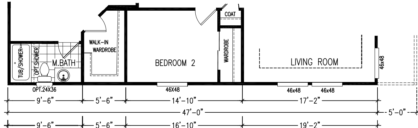
OPTIONAL 2-BEDROOM LAYOUT
