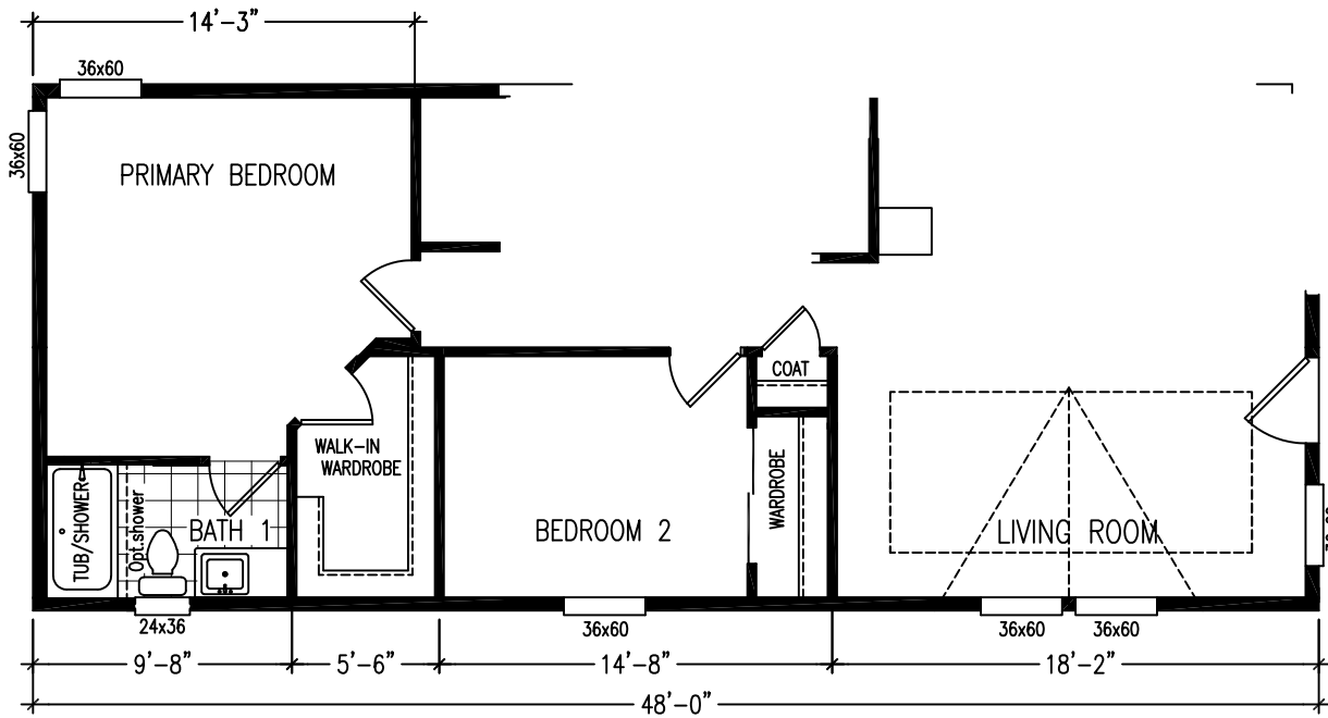
OPTIONAL 2-BEDROOM LAYOUT
